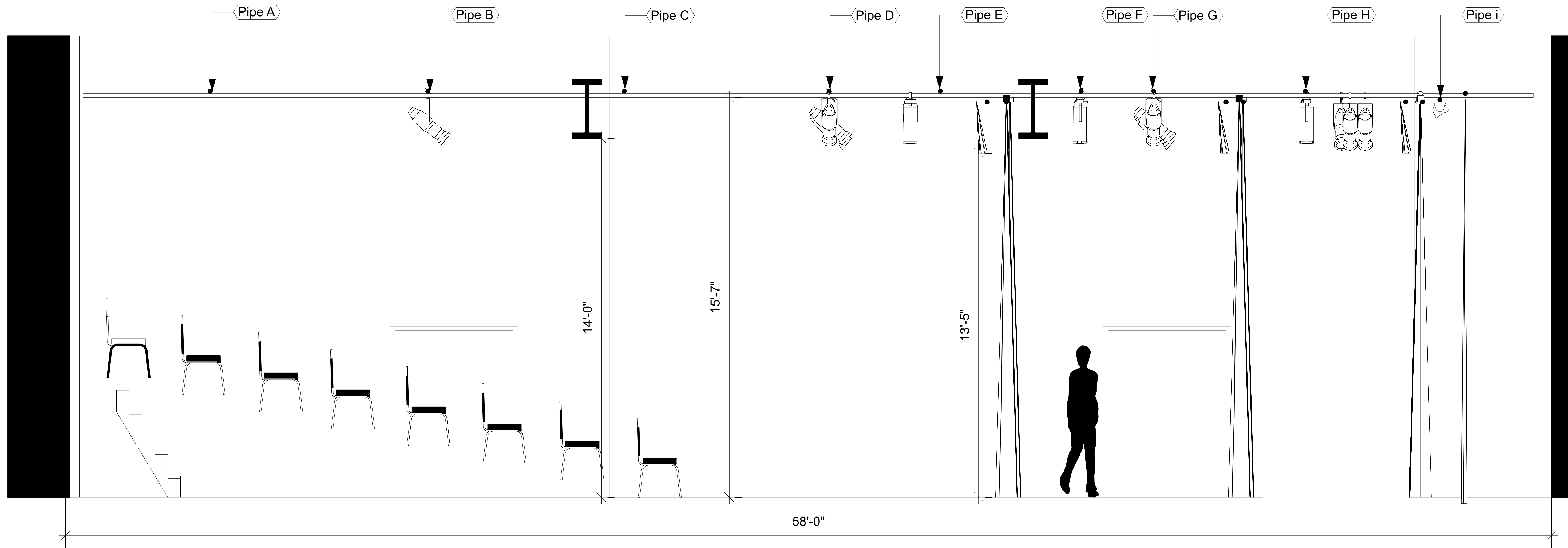
2 Section Scale: 1/2" = 1'-0"
